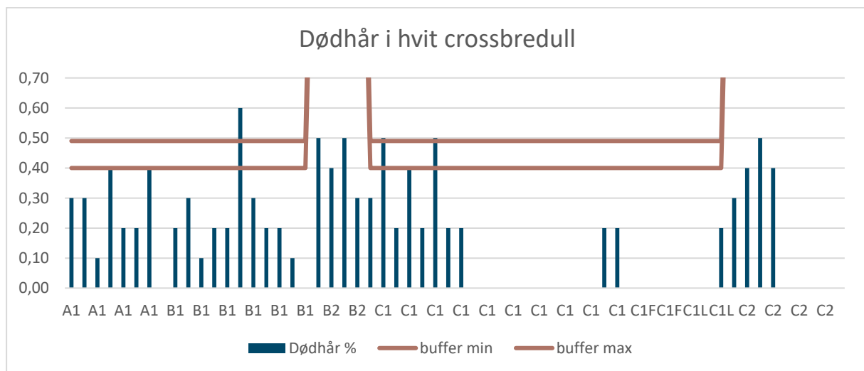
Figur 3: dødthår (i prosent) i hvit crossbredull (A1, B1, B2, C1, C1 fin, C1 lam og C2) Buffergrensa for andresortering er 2 %. Ingen prøver er i nærheten av den verdien
